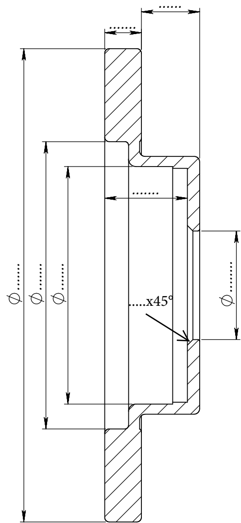
SEZIONE A-A
